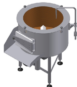
Машины для обезглавливания рыбы
